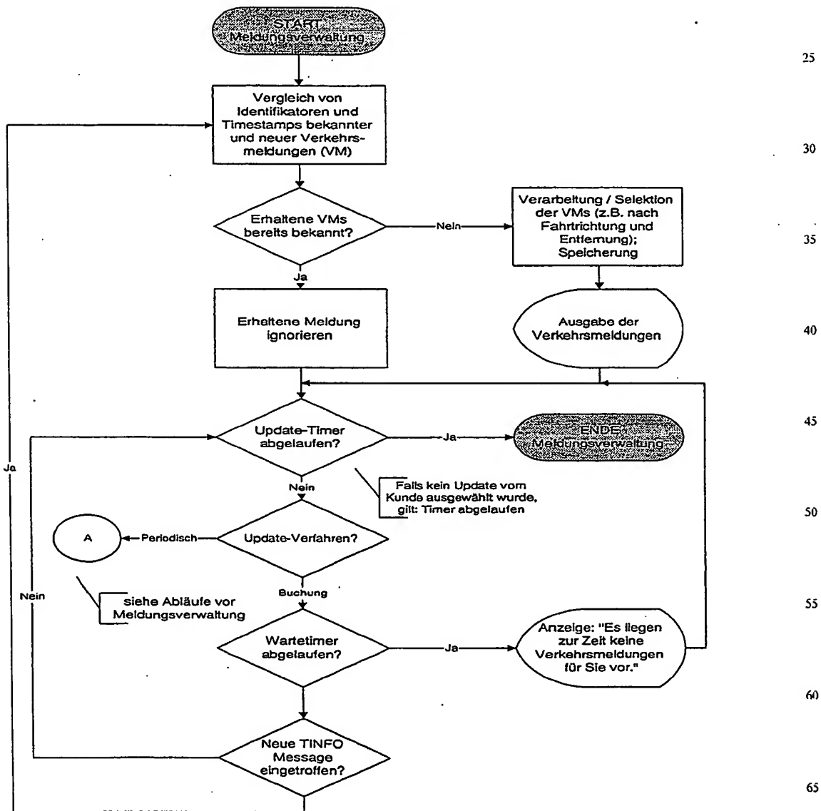
Abb. 7.1: Meldungsverwaltung
